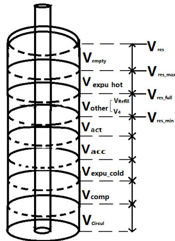
图1 油箱各容积示意图
