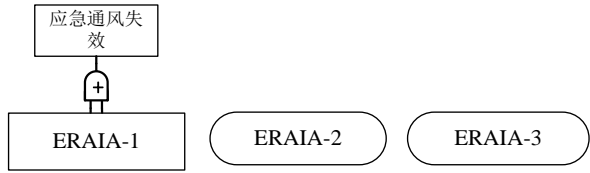
(b) 应急冲压空气作动器故障逻辑
