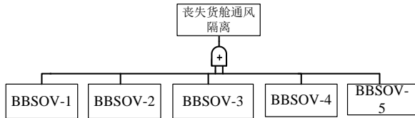
(d) 货舱关断活门故障逻辑
