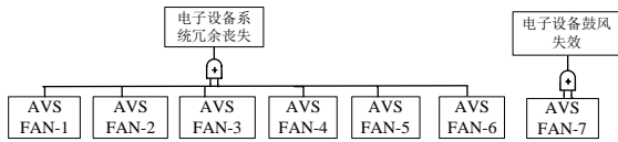
(f) 电子设备风扇故障逻辑
