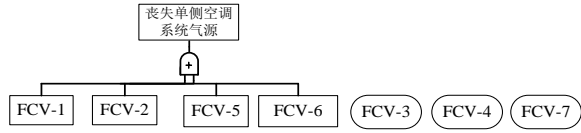
(a) 流量控制活门故障逻辑
