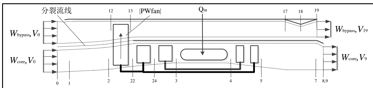
图1 分排涡扇发动机示意图
