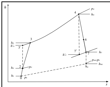
图2 热力循环焓—熵图
