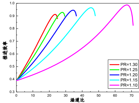
(a) 外涵压比 1.0~1.3 条件下
