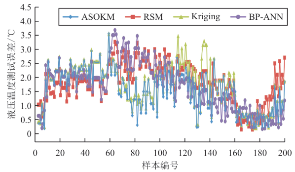
图6 液压系统监测误差结果
