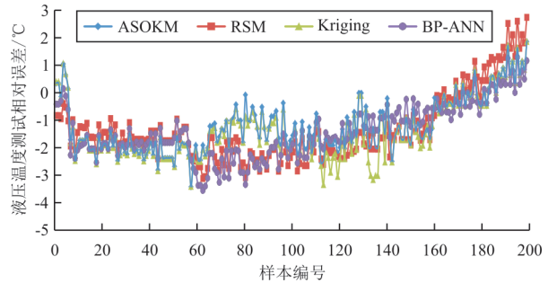
图7 液压系统监测相对误差结果
